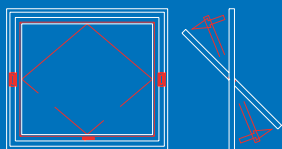
Ventana pivotante
